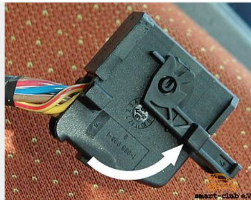
Der Kombiinstrumentstecker
